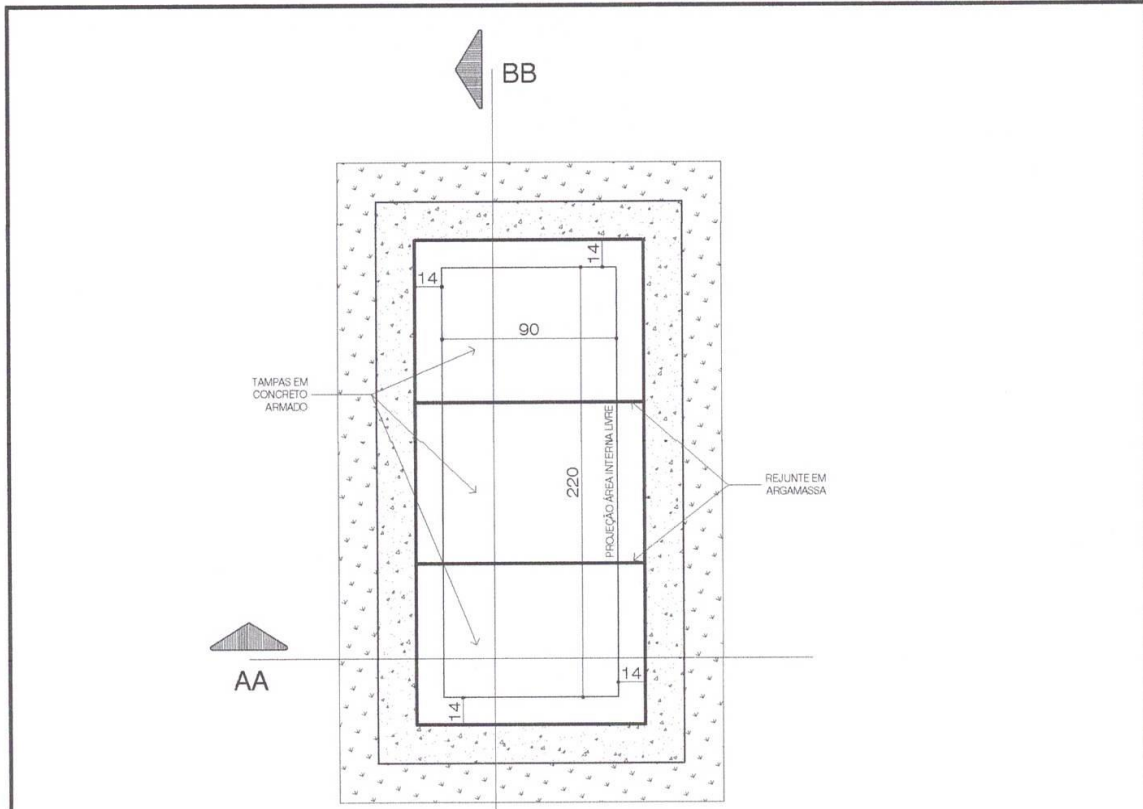
PLANTA - SEPULTURA ESCALA S/E - MEDIDAS EM CENTIMETROS
