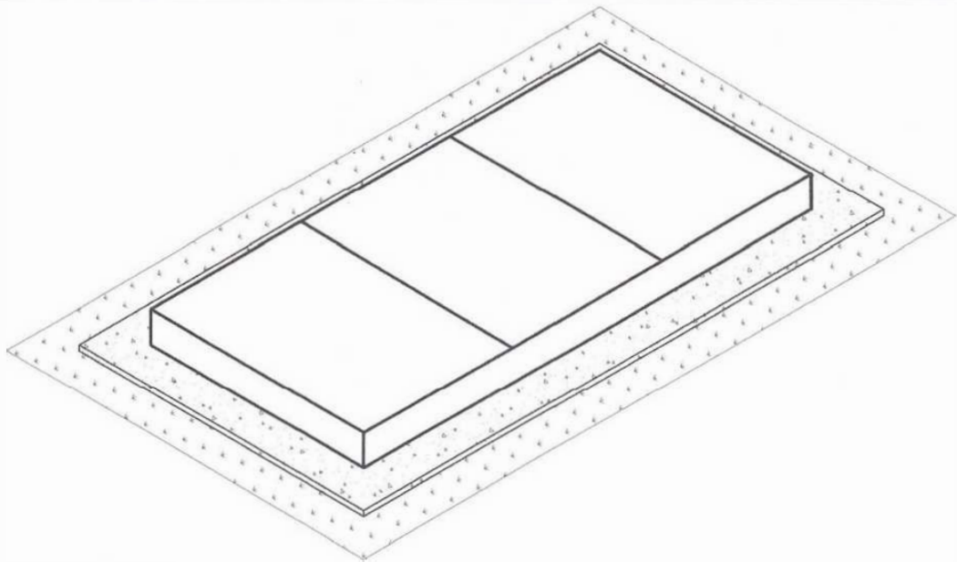
PERSPECTIVA DA SEPULTURA ESCALA S/E - MEDIDAS EM CENTIMETROS
