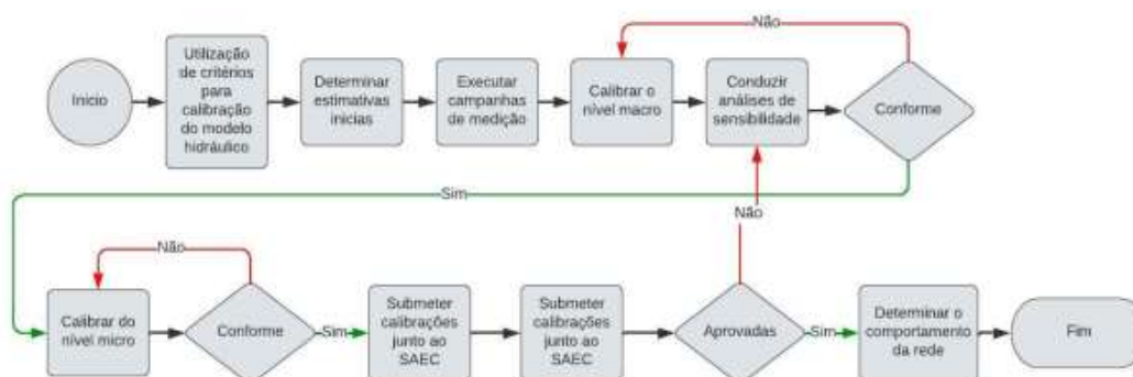
Figura 0.1. Calibração do modelo hidráulico
