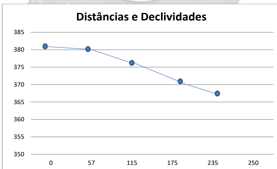
Figura 39 - Perfil longitudinal do canal 4 - (sem escala)
