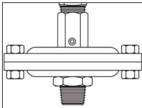
Figura 1: Diafragma a ser fornecido com o manômetro.
