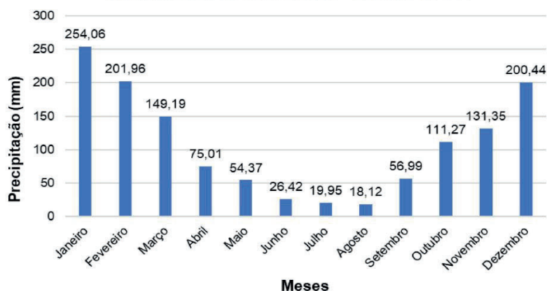
Figura 4: Precipitação Média Mensal no período de 1960 a 2021
