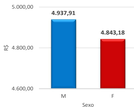
REMUNERAÇÃO MÉDIA
