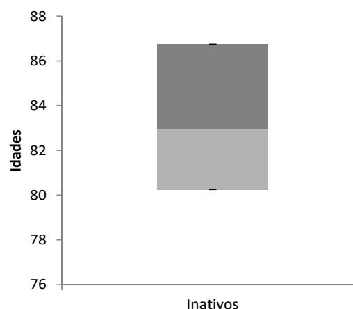
BOXPLOT INATIVOS
