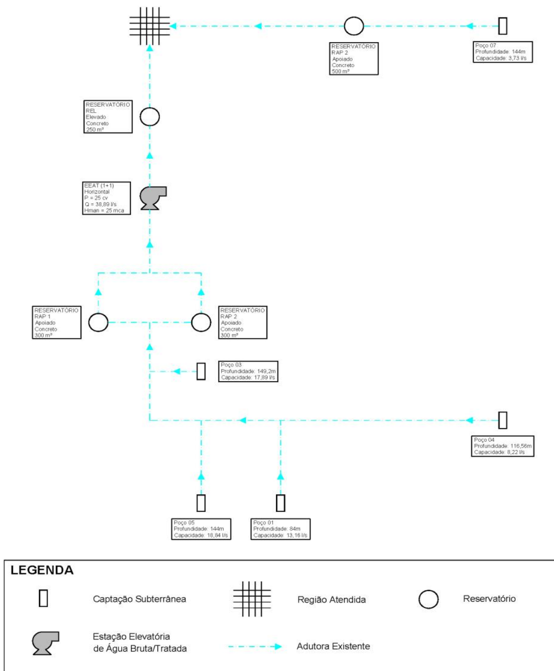
Figura 6 – Croqui do Sistema de Abastecimento de Água Existente da Sede Urbana
