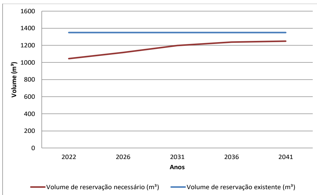
Gráfico 8.1 - Volume de Reservação Necessário (m³) x Volume de Reservação Atual (m³)
