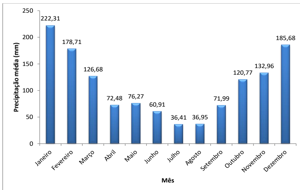
Gráfico 3.1 – Precipitação Média Mensal no Período de 1936 a 2021, Estação D7-001
