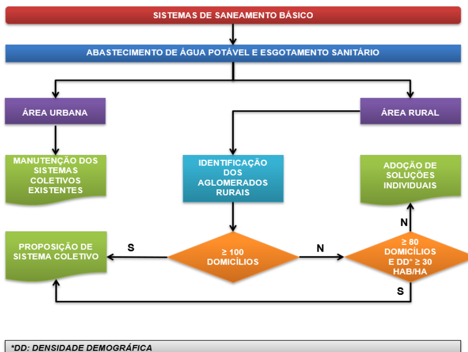
Figura 3 – Fluxograma da Metodologia Aplicada para Definição das Soluções (Coletiva ou Individual)
