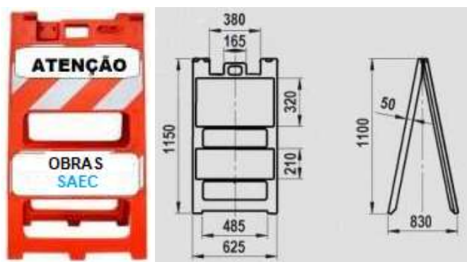
Figura 3 – Cavalete plástico de 1,15m (referente ao item 3)
