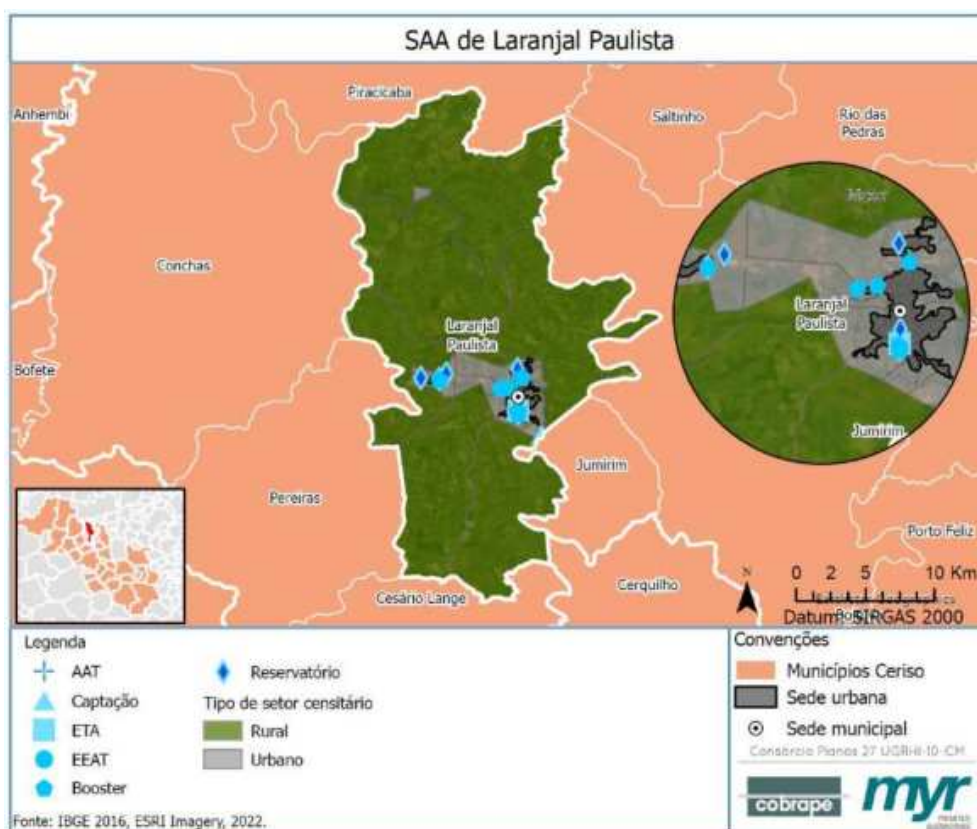
Figura 5-2 – Estruturas do SAA de Laranjal Paulista na área urbana e rural
