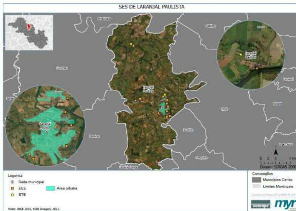
Figura 5-1 – Principais Estruturas do Sistema de Esgotamento Sanitário de Laranjal Paulista/SP.
