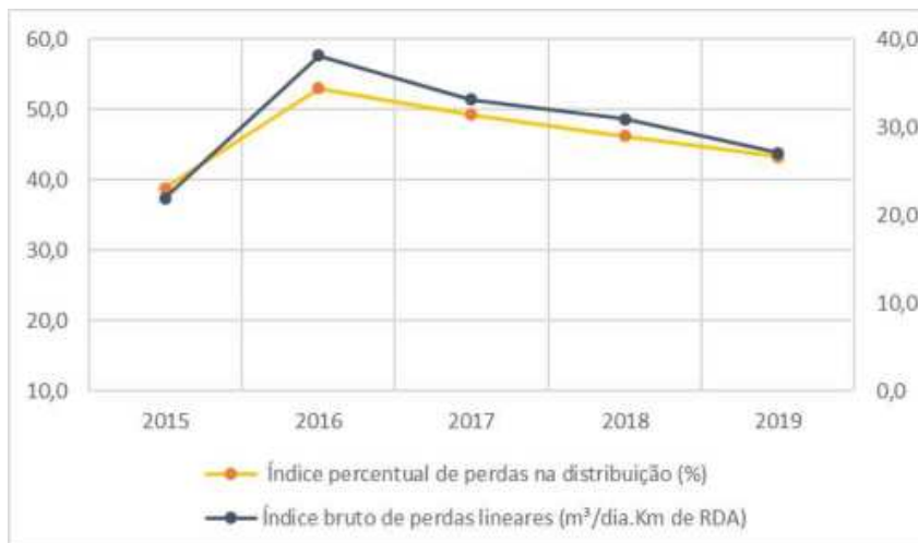
Figura 4-22 – Comparativo entre os índices de perda do SAA de Laranjal Paulista/SP
