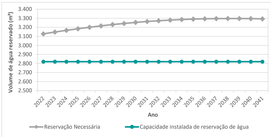
Figura 5-5 - Reservação necessária e capacidade instalada para sistemas coletivos
