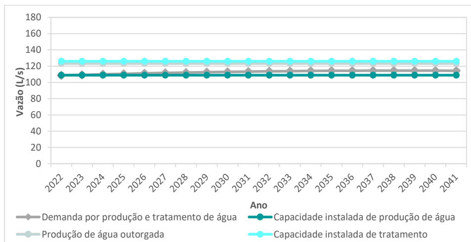
Figura 5-4 - Demanda total e vazão de produção e tratamento existentes para coletivos
