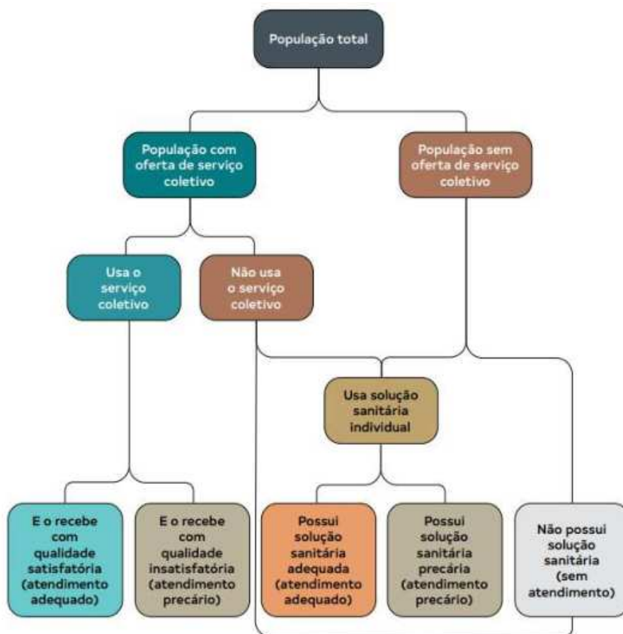
Figura 5-16 – Fluxograma de soluções sanitárias
