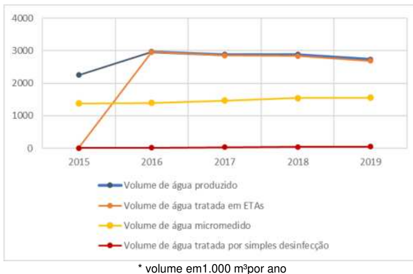
Figura 4-21 – Comparativo entre os volumes operacionais entre 2015 e 2019 do SAA de Laranjal Paulista/SP
