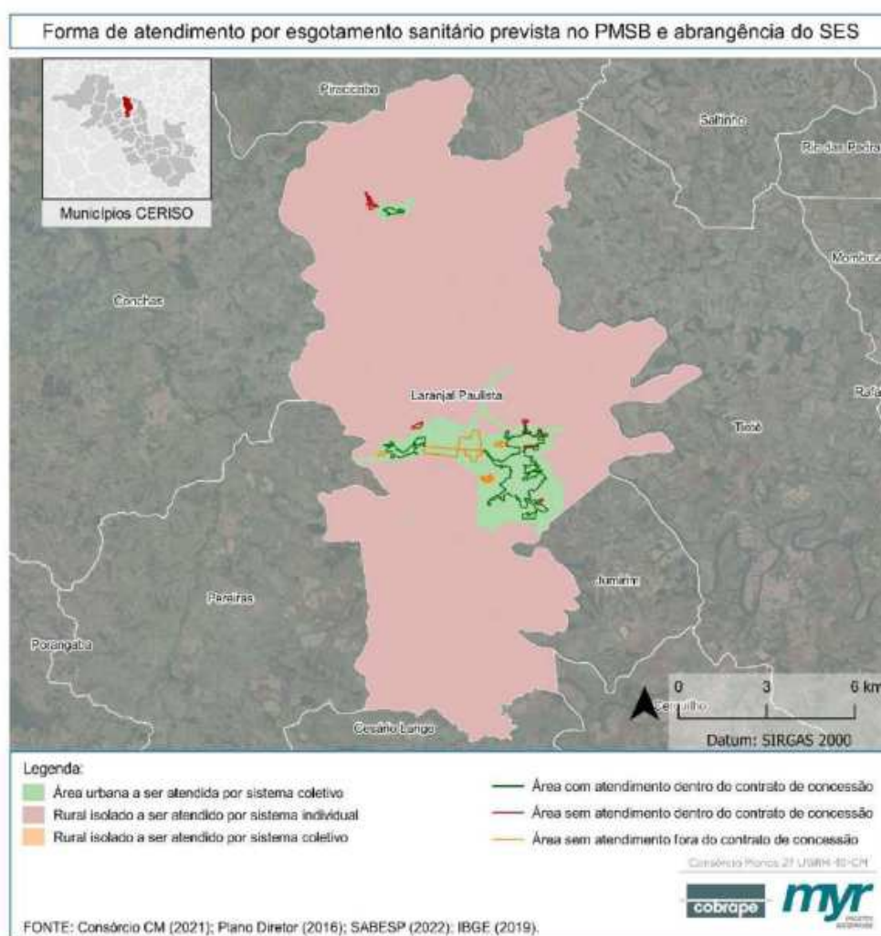
Figura 5-7 – Previsão de atendimento por soluções individuais e coletivas de esgotamento sanitário conforme ordenamento do zoneamento municipal
