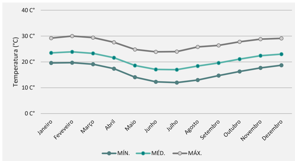
Figura 3-41 – Temperatura máxima, média e mínima em graus na estação Sorocaba
