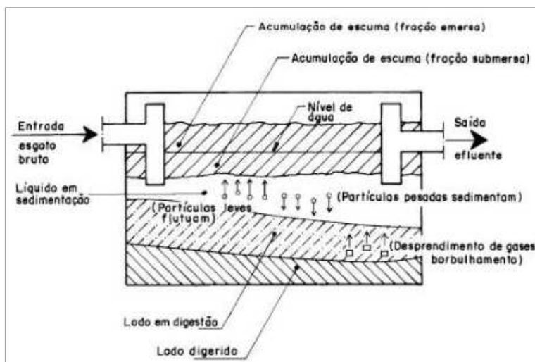
Figura 5-17 – Funcionamento de um tanque séptico.
