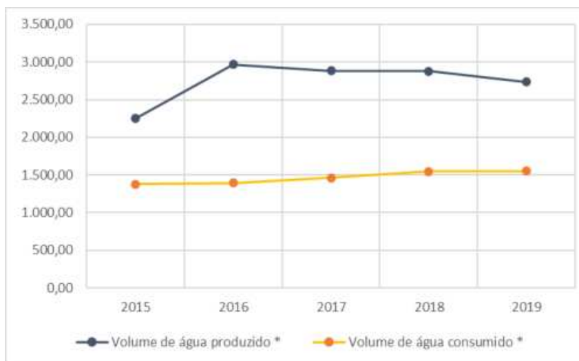
Figura 4-20 – Comparativo entre os volumes produzido x consumido entre 2015 e 2019 do SAA de Laranjal Paulista/SP
