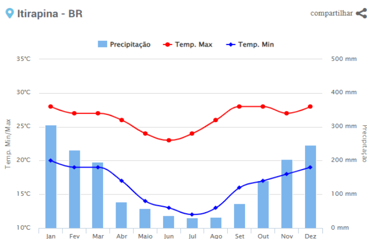
Figura 2 – Pluviometria (Fonte: https://www.climatempo.com.br/climatologia/2355/itirapina-sp )
