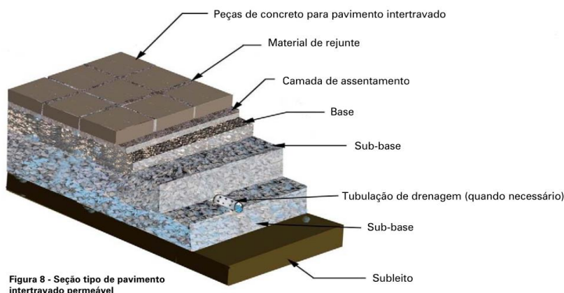
Figura 85 - Seção tipo de pavimento intertravado permeável
