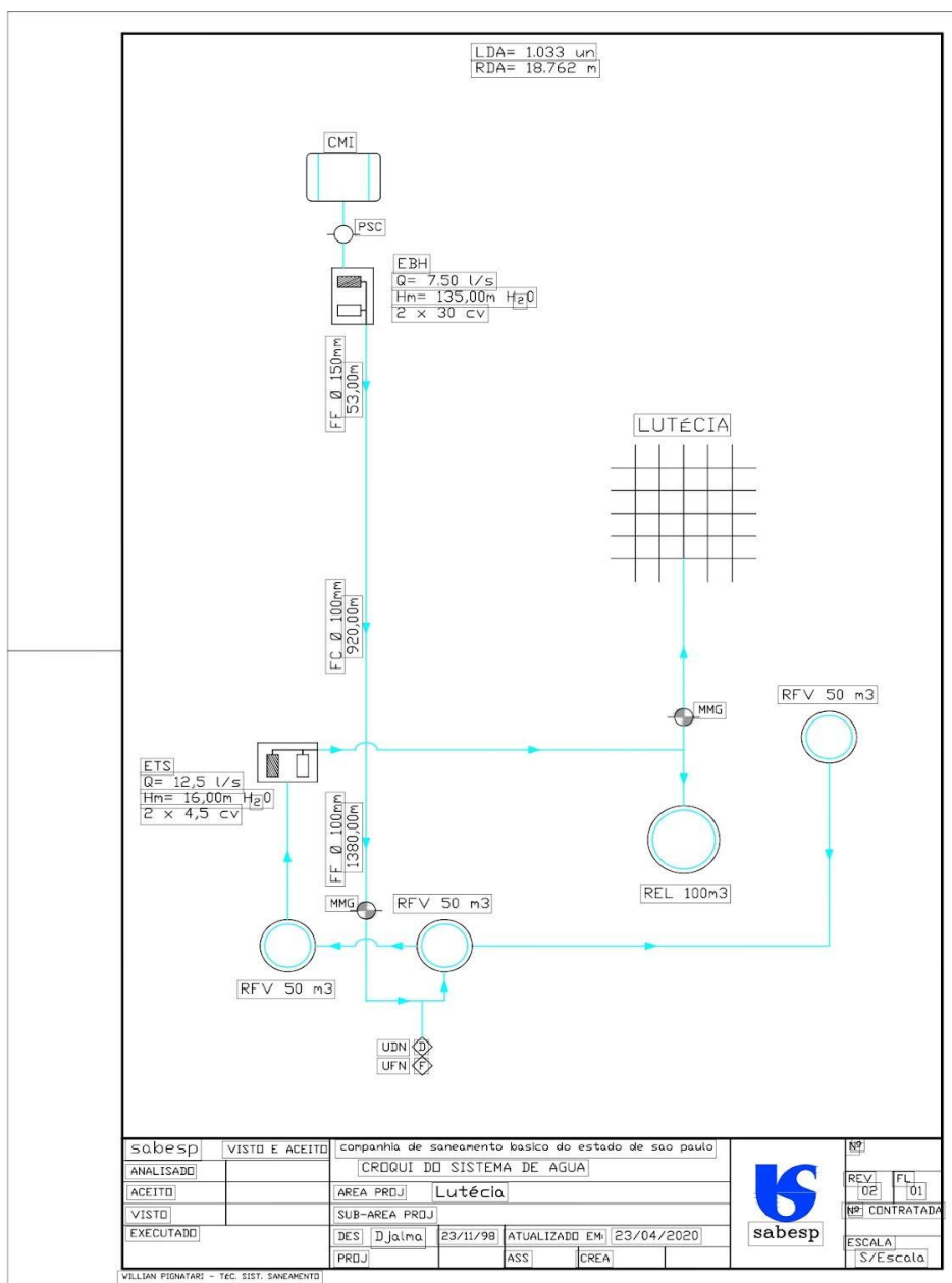
Figura 71 - Croqui do sistema de água
