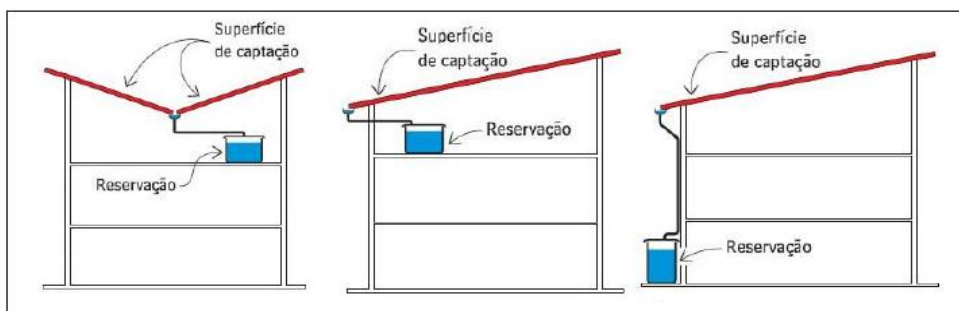
Figura 86 - Esquema de soluções de captação e alimentação do reservatório de águas pluviais
