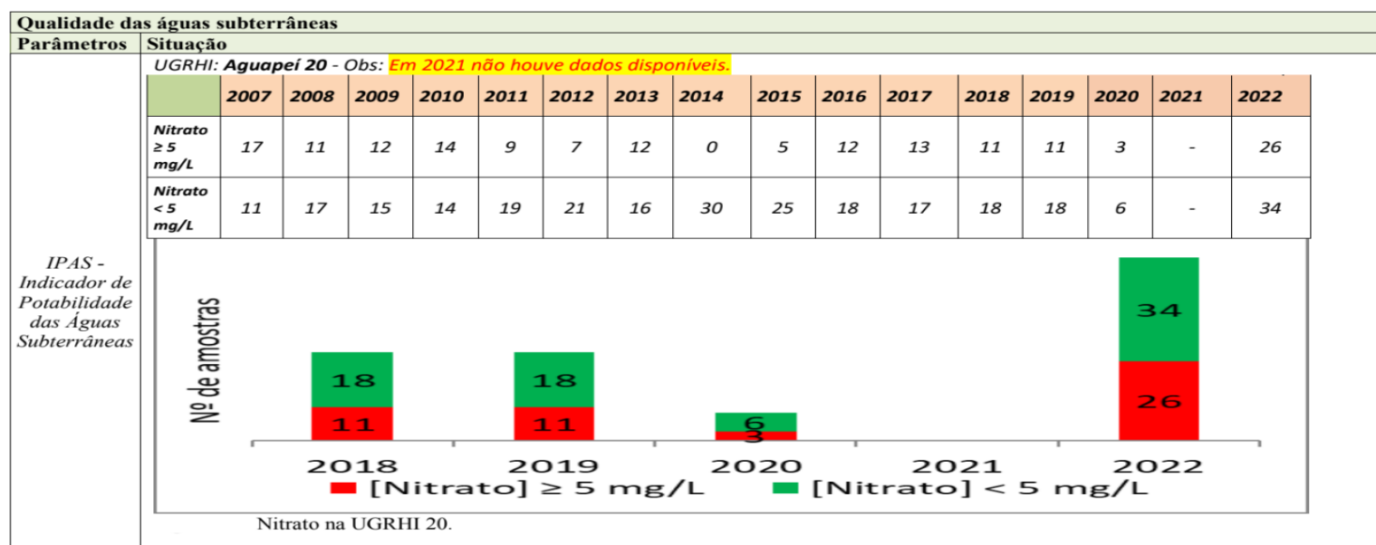
Figura 57 - Quadro Síntese da Potabilidade das Águas Subterrâneas (IPAS) para as UGRHI 20
