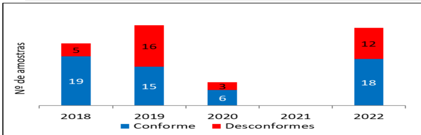
Classificação das águas subterrâneas, quanto à potabilidade na UGRHI 20
