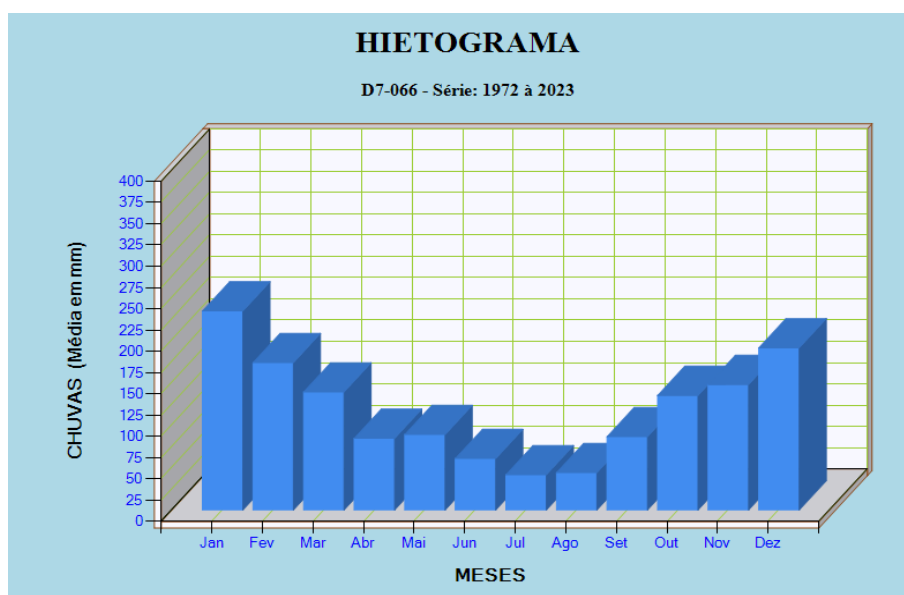
Figura 16 - Pluviograma (Estação D7-066 - bairro Tabajara - rural)
