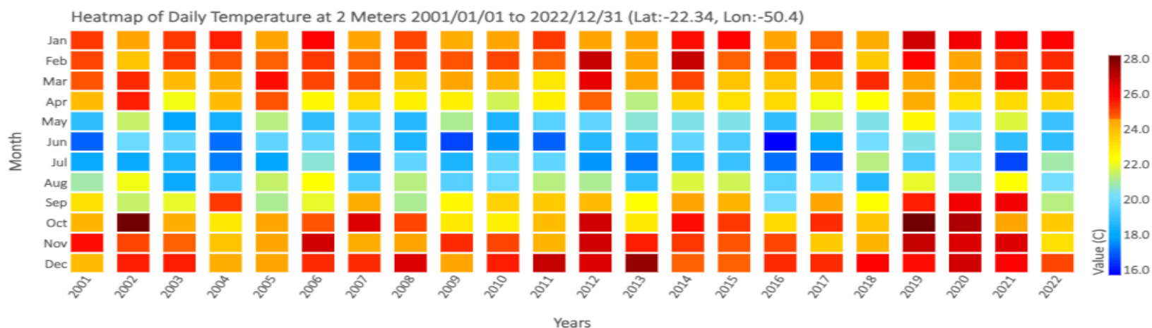
Figura 13 - Gráfico de Temperaturas Médias em Lutécia (de 2001 a 2022)
