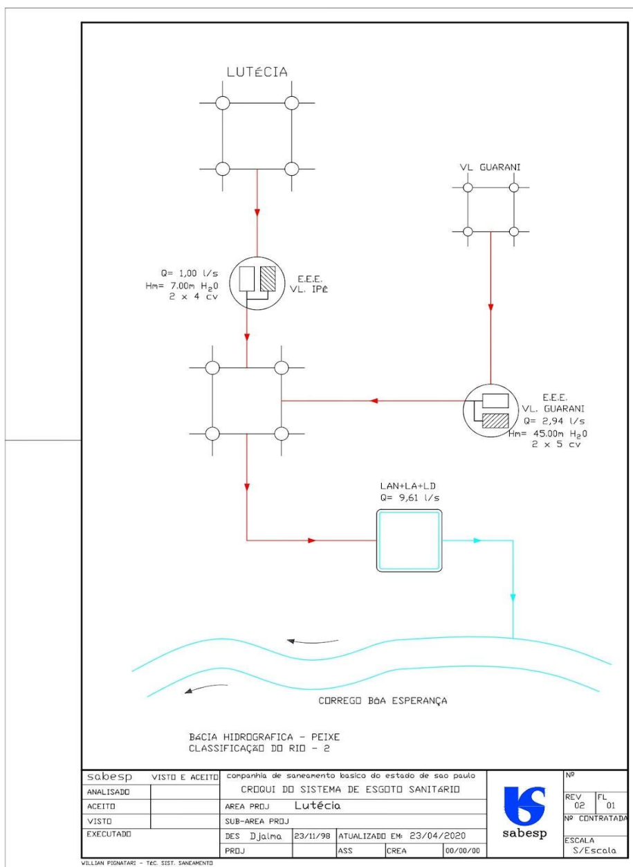
Figura 72 - Croqui do sistema de esgoto sanitário
