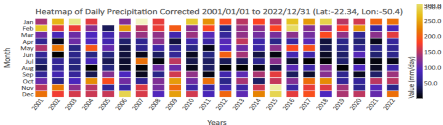
Figura 14 - Gráfico de Precipitação Média em Lutécia (de 2001 a 2022)
