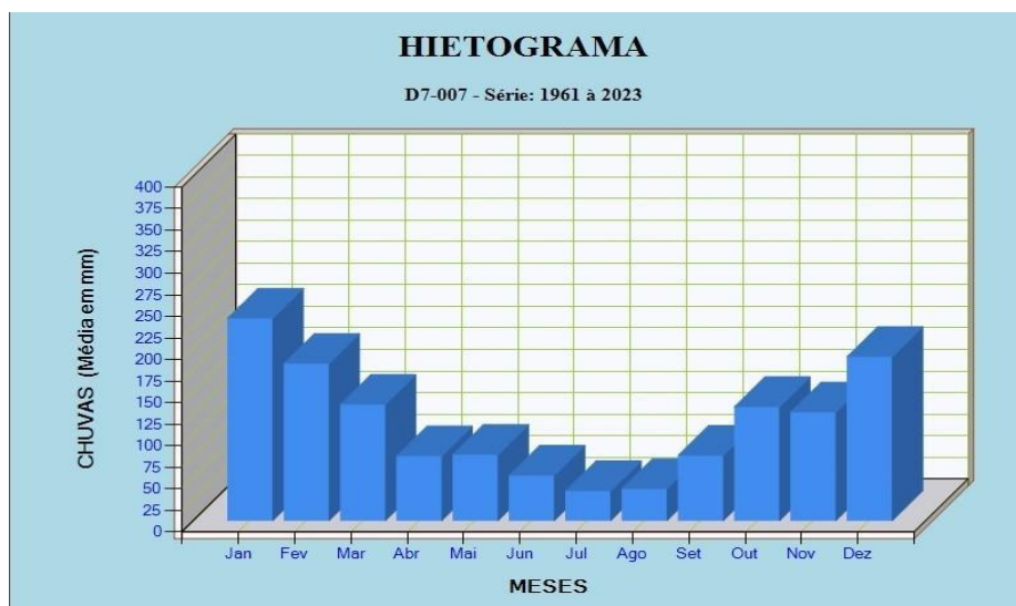
Figura 15 - Pluviograma (Estação D7-007 - cidade)
