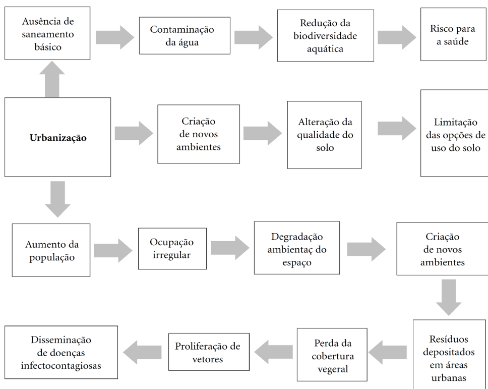
Figura 49 - Diagrama de Interação Urbanização-Saneamento-Saúde
