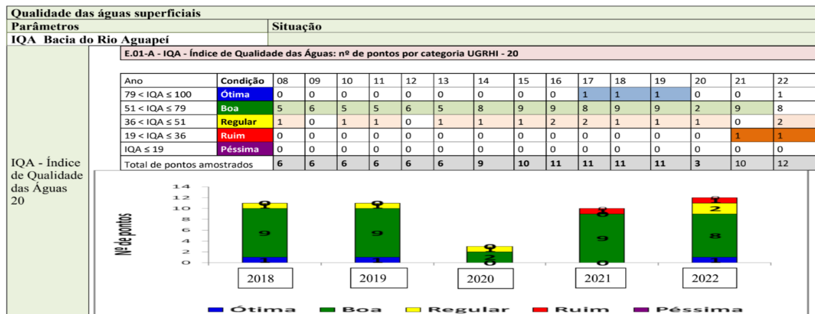
Figura 52 - Quadro Síntese da Qualidade das Águas (IQA) para a UGRHI 20
