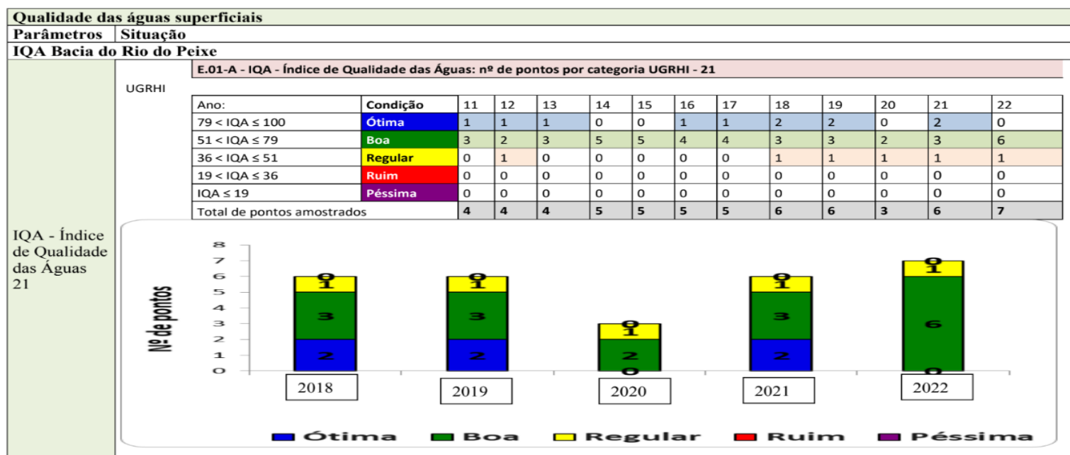
Figura 53 - Figura 62 - Quadro Síntese da Qualidade das Águas (IQA) para a UGRHI 21
