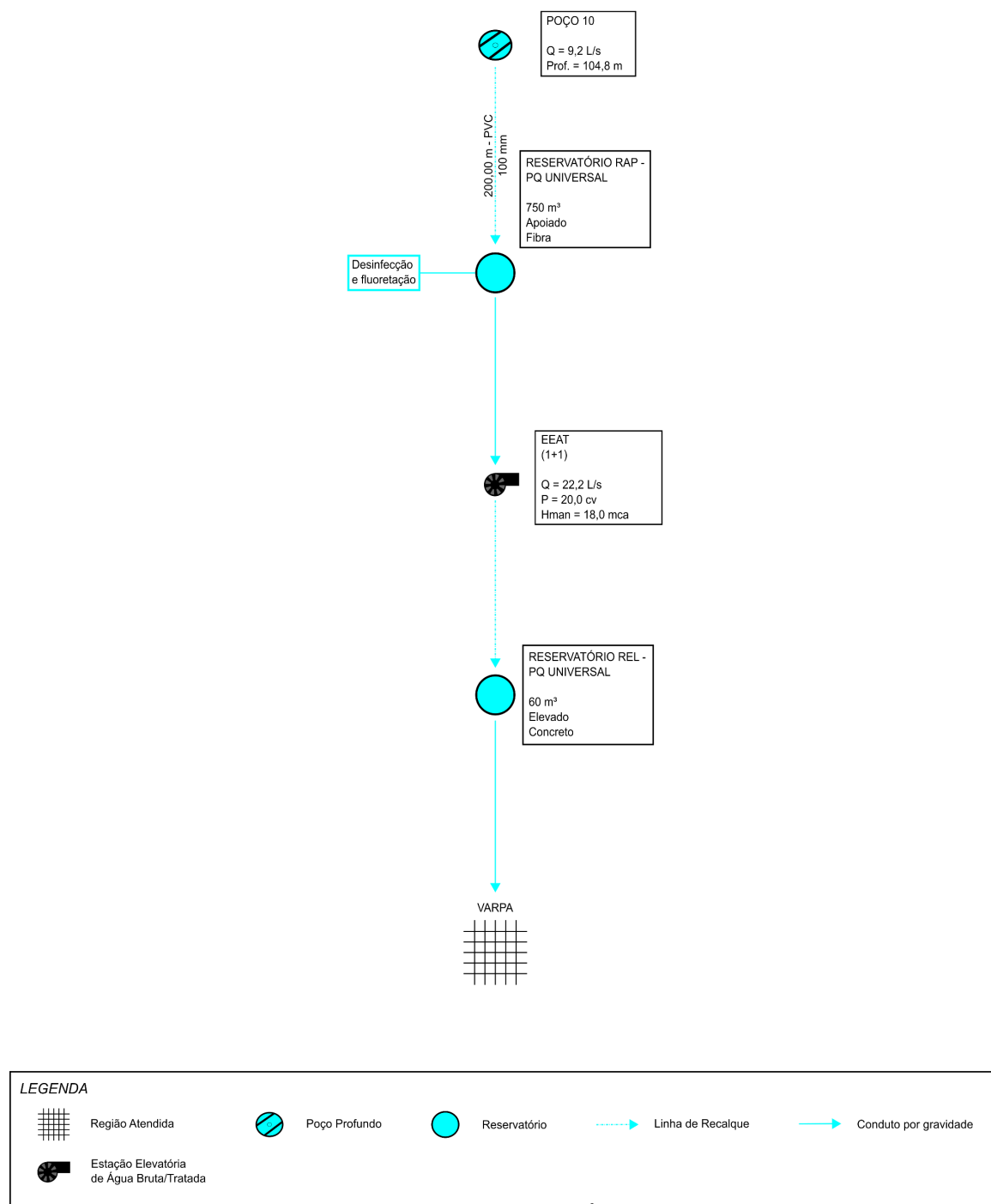
Figura 02 – Croqui do Sistema de Abastecimento de Água Parque Universitário
