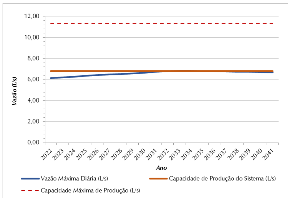
Figura 0.7 – Demandas Máximas Diárias (L/s) X Vazão Captada (L/s) – SAA Parque Industrial
