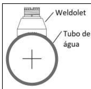
Figura 2: Desenho esquemático do Weldolet instalado.
