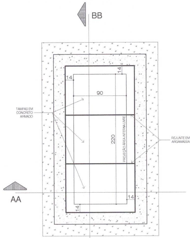
PLANTA - SEPULTURA ESCALA S/E - MEDIDAS EM CENTIMETROS
