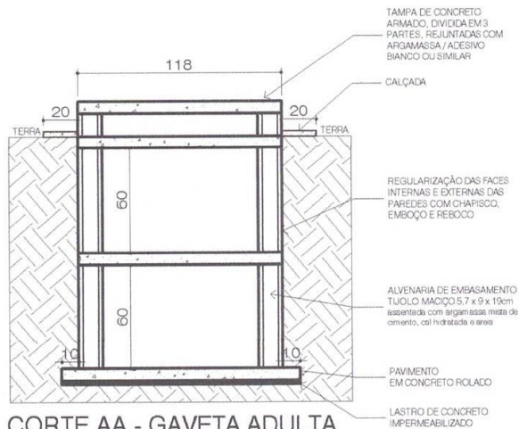
CORTE AA - GAVETA ADULTA ESCALA S/E - MEDIDAS EM CENTIMETROS
