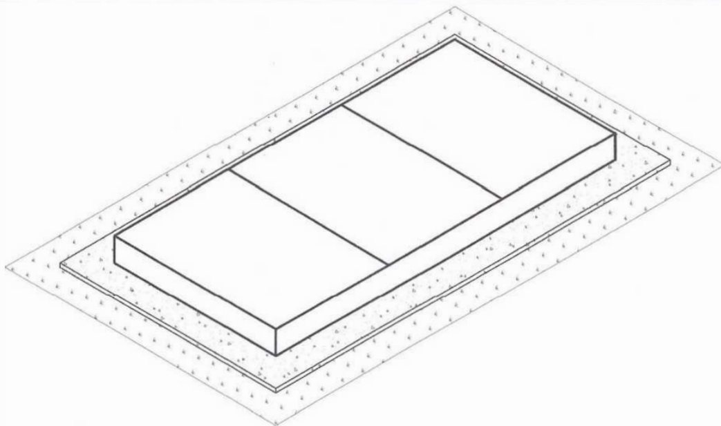
PERSPECTIVA DA SEPULTURA ESCALA S/E - MEDIDAS EM CENTIMETROS
