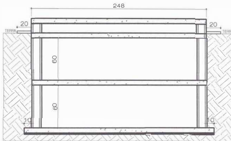
CORTE BB - GAVETA ADULTA ESCALA S/E - MEDIDAS EM CENTIMETROS
