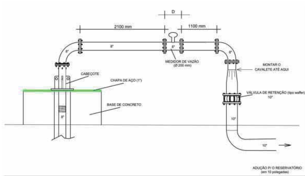
Figura 4-5: Barrilete de produção
