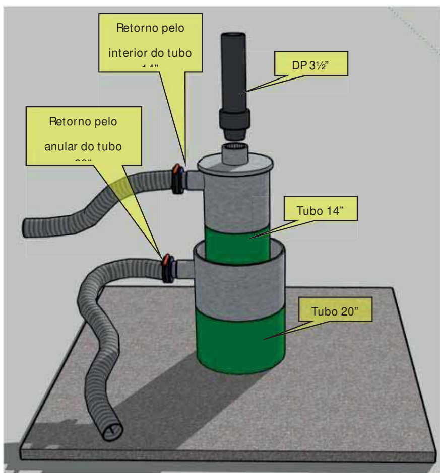
Figura 4-2: Cabeça para circulação de lama e cimentação
