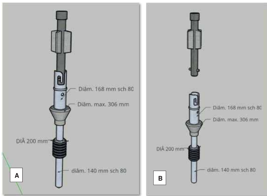
Figura 4-1: Desenho esquemático do obturador: Com engate baioneta acoplado (A) e desacoplado (B)
