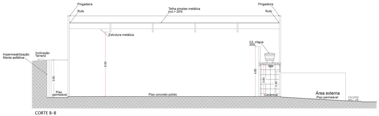
CORTE B-B
