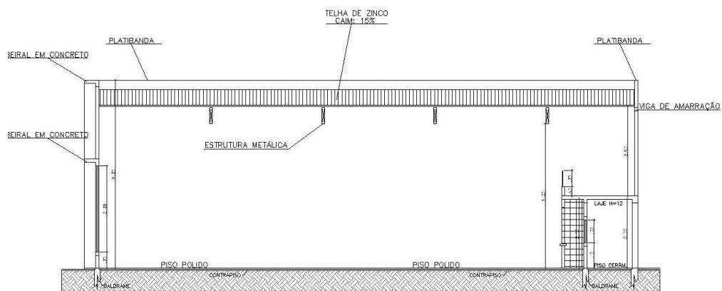
CORTE A ESCALA 1/100
