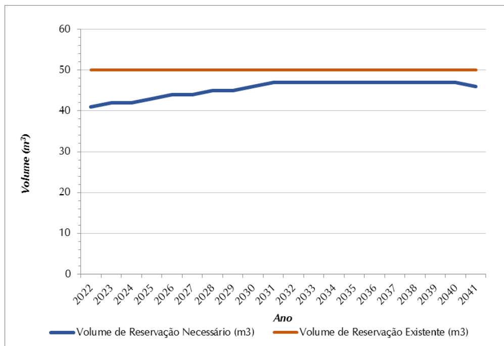
Figura 0.14 - Volume de Reservação Necessário (m³) x Volume de Reservação Atual (m³) – SAA Varpa
