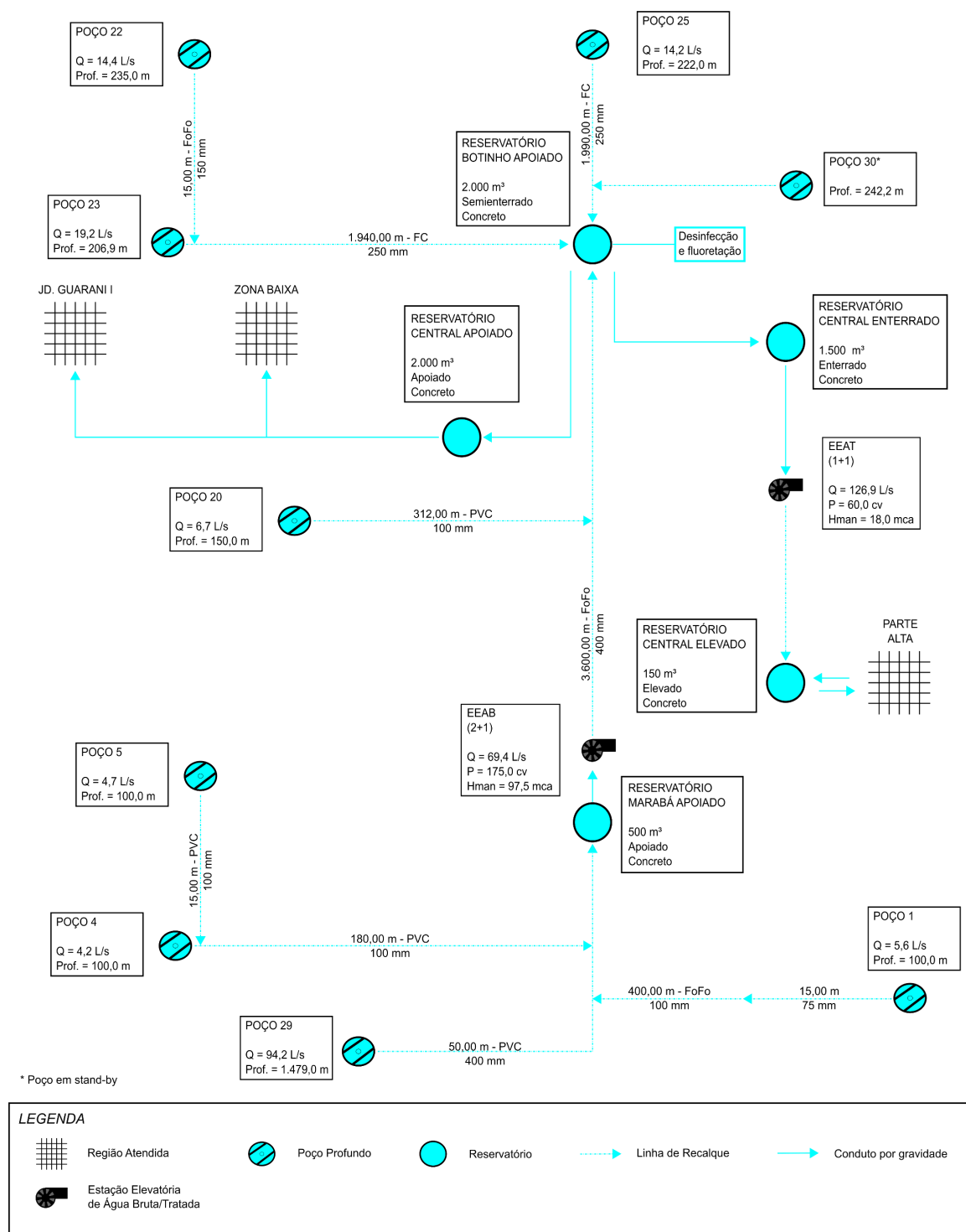
Figura 0.1 – Croqui do Sistema de Abastecimento de Água Central Fonte: SABESP, 2021.
