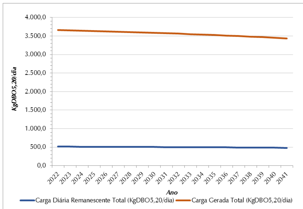
Figura 0.16 - Evolução de Cargas Orgânicas (Kg DBO 5,20 /Dia) – SES Sede
