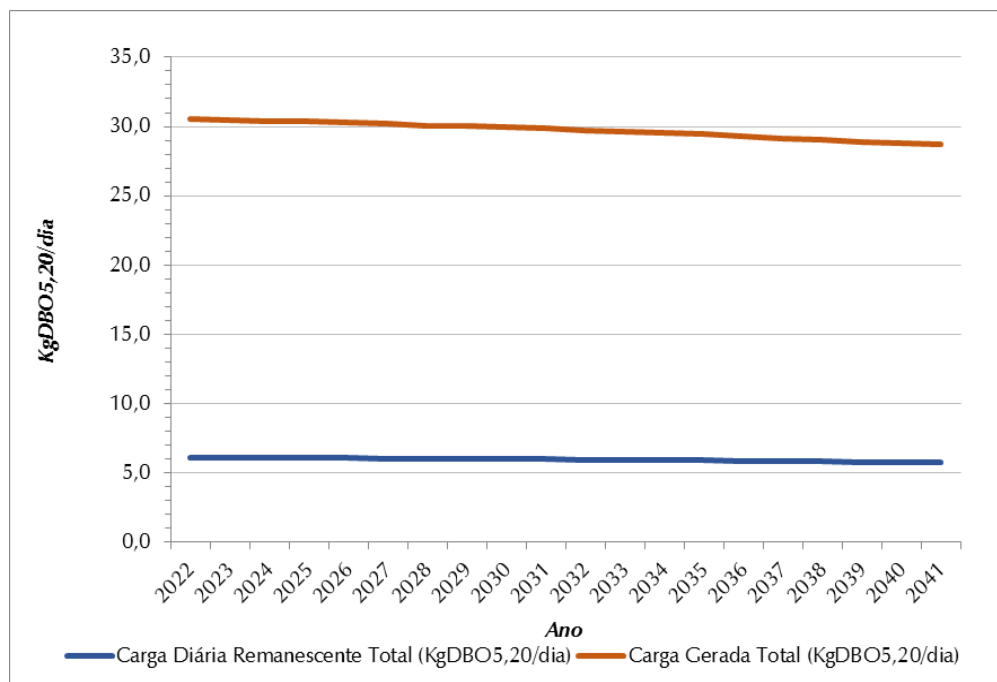
Figura 0.18 - Evolução de Cargas Orgânicas (Kg DBO 5,20 /Dia) – SES Parnaso
