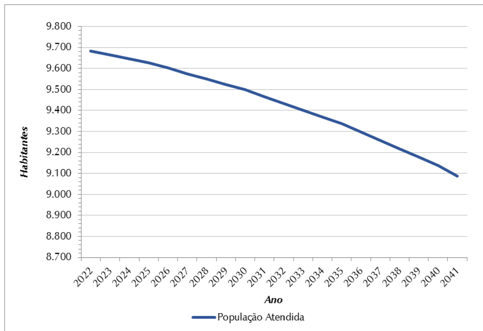
Figura 0.5 – Evolução da População Atendida (hab) – SAA Vila Formosa
