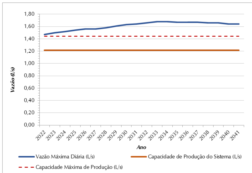
Figura 0.9 – Demandas Máximas Diárias (L/s) X Vazão Captada (L/s) – SAA Parnaso
