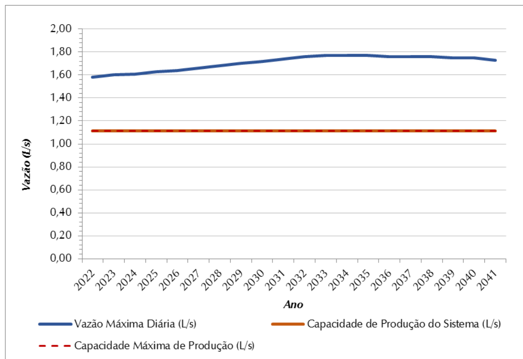
Figura 0.11 – Demandas Máximas Diárias (L/s) X Vazão Captada (L/s) – SAA Universo
