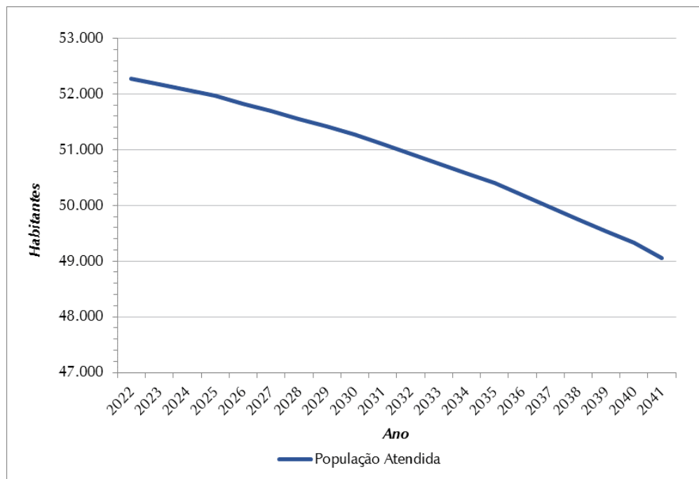
Figura 0.3 – Evolução da População Atendida (hab) – SAA Central
