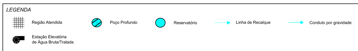
Figura 0.3 – Croqui do Sistema de Abastecimento de Água Vila Formosa Fonte: SABESP, 2021
