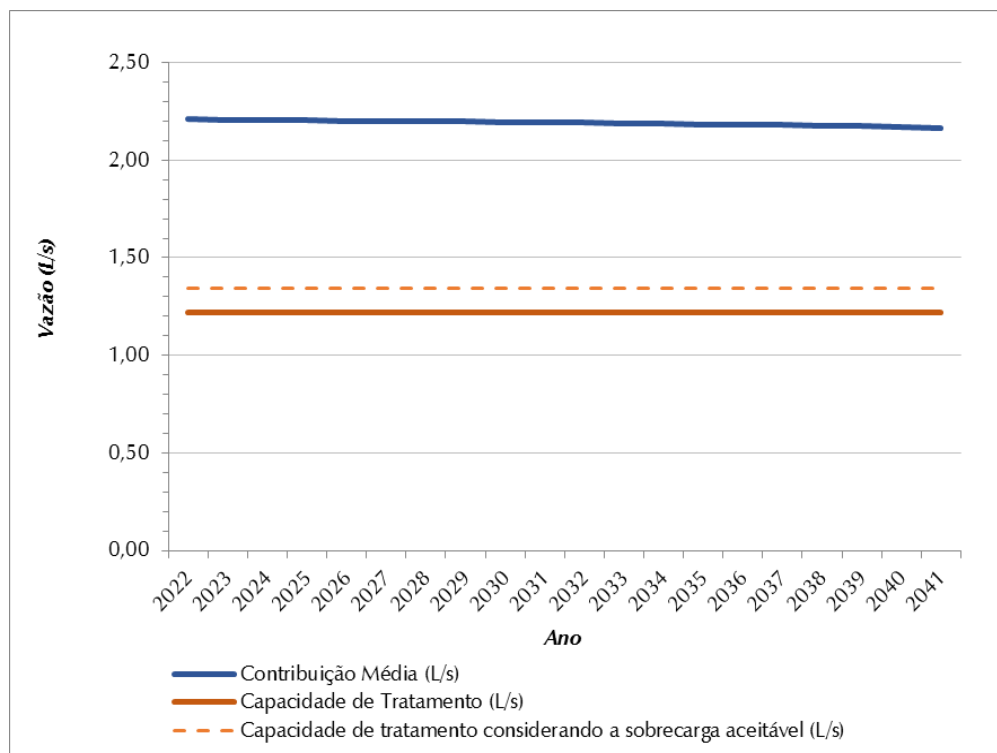
Figura 0.21 – Contribuição Média Total (L/s) x Capacidade de Tratamento de Esgoto (L/s) – SES Varpa
