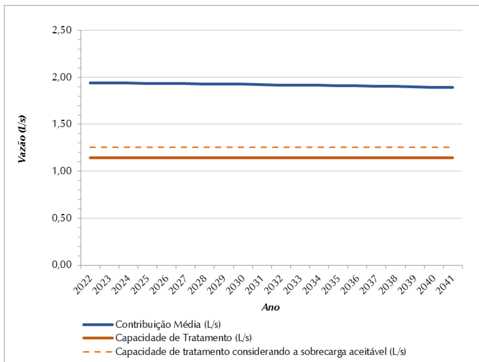
Figura 0.17 – Contribuição Média Total (L/s) x Capacidade de Tratamento de Esgoto (L/s) – SES Parnaso
