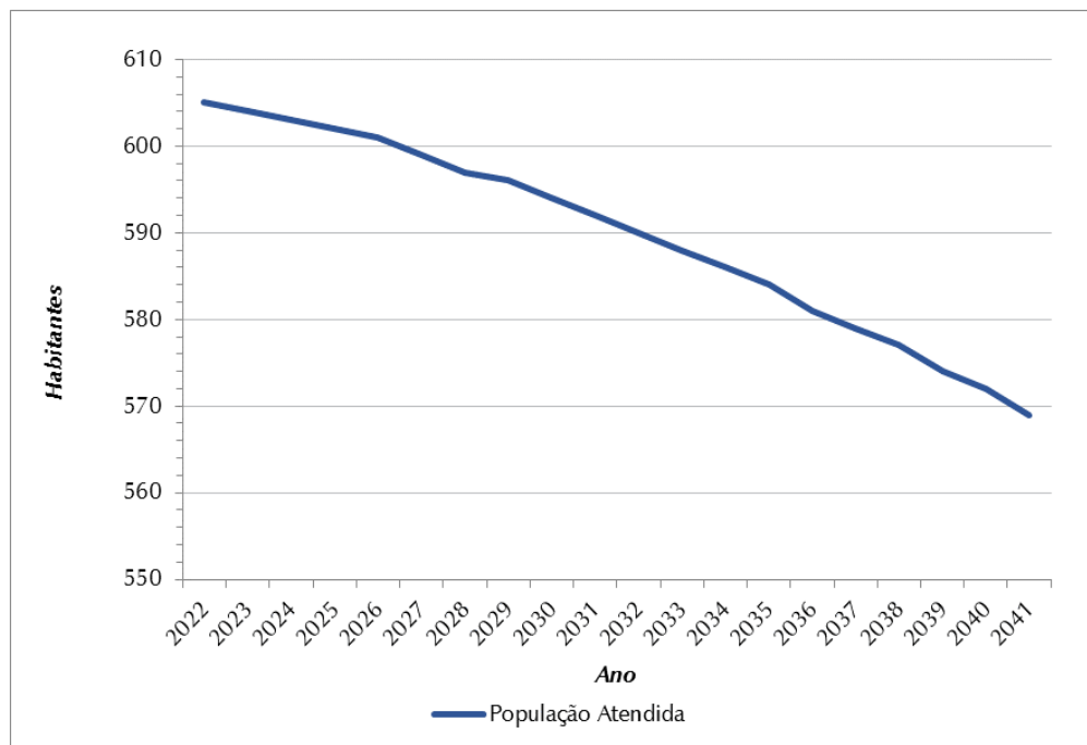
Figura 0.9 – Evolução da População Atendida (hab) – SAA Varpa
