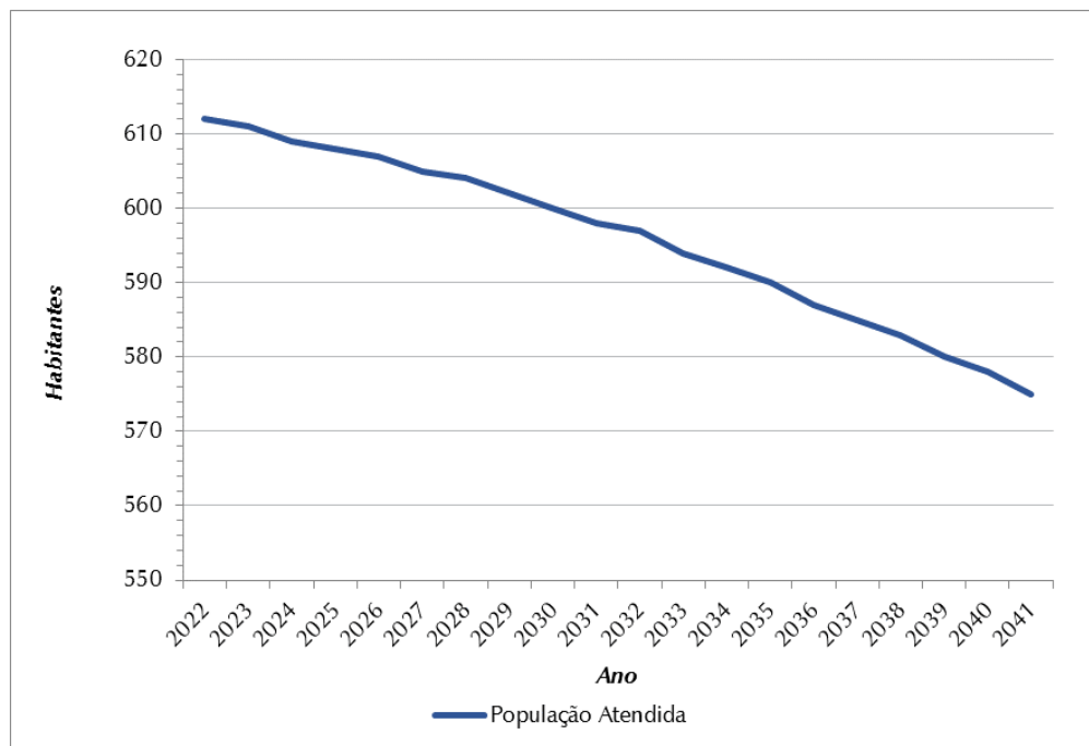
Figura 0.8 – Evolução da População Atendida (hab) – SAA Universo
