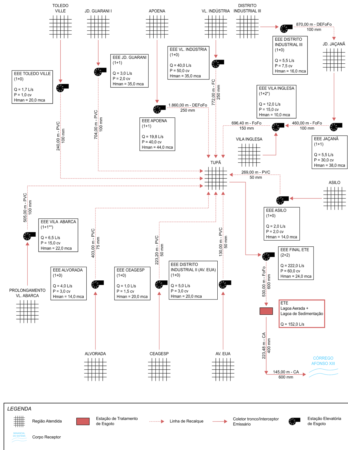
Figura 08 – Croqui do Sistema de Esgotamento Sanitário da Sede Fonte: SABESP, 2021.
