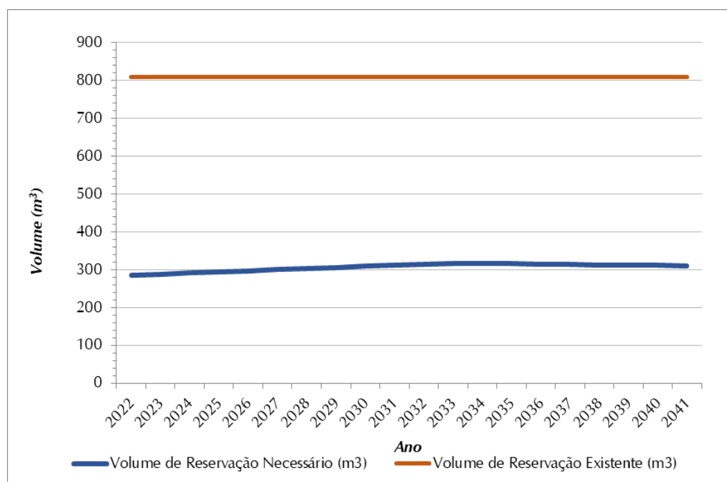
Figura 0.4 - Volume de Reservação Necessário (m³) x Volume de Reservação Atual (m³) – SAA Parque Universitário
