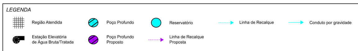
Figura 0.6 – Croqui das intervenções propostas para o sistema de abastecimento de água Universitário
