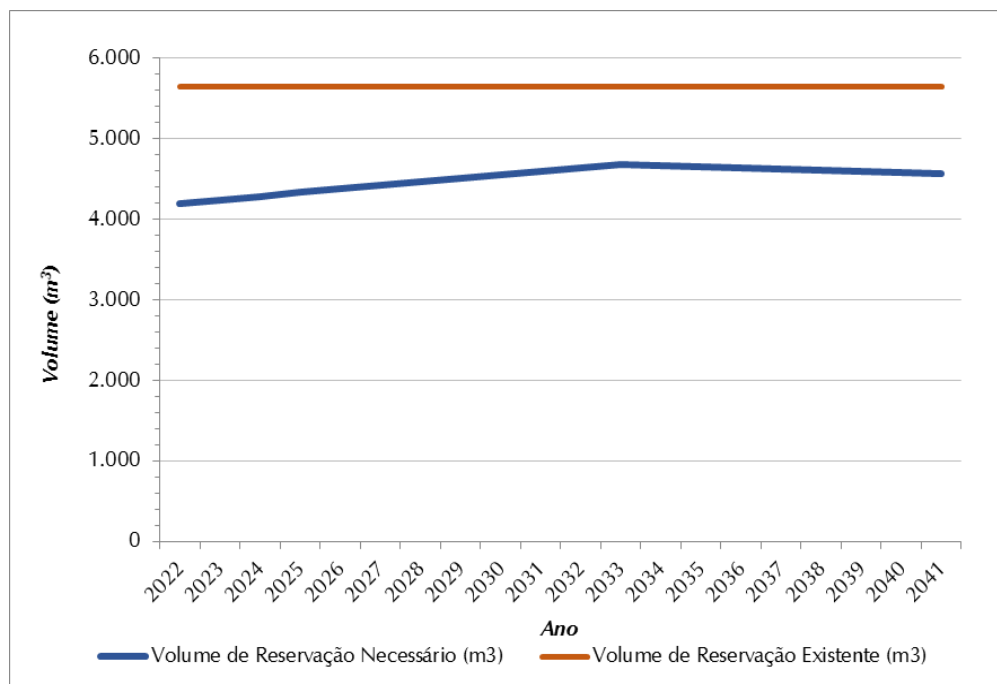
Figura 0.2 - Volume de Reserva Necessário (m³) x Volume de Reserva Atual (m³) – SAA Central
