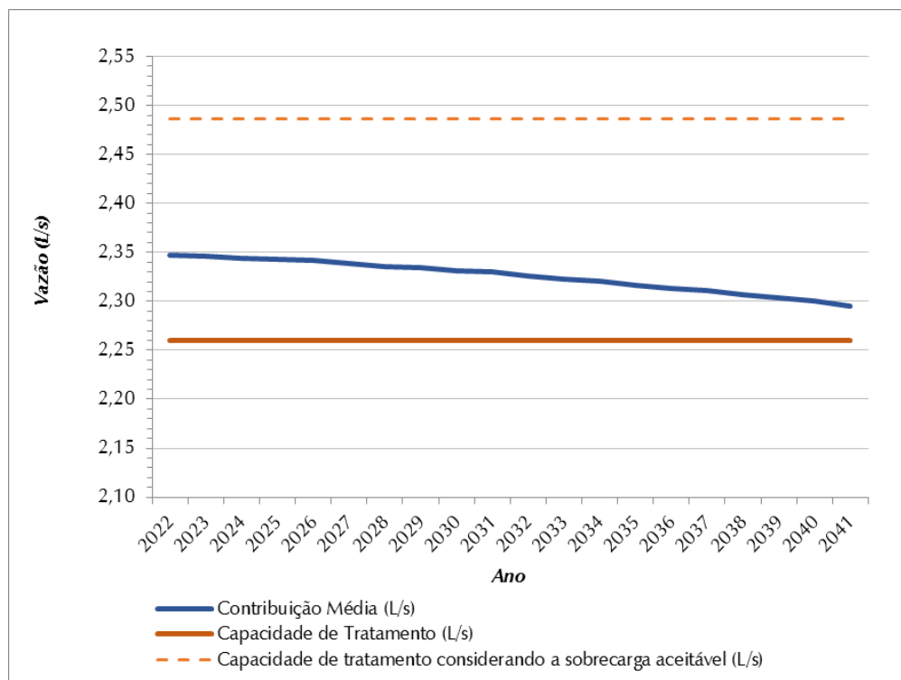
Figura 0.19 – Contribuição Média Total (L/s) x Capacidade de Tratamento de Esgoto (L/s) – SES Universo
