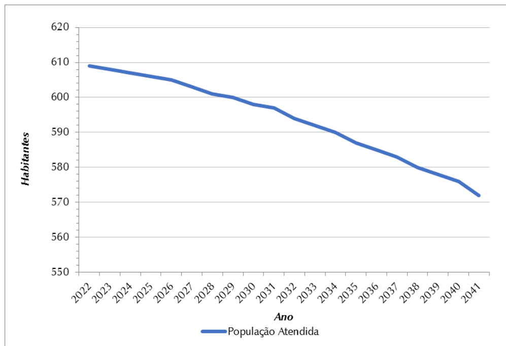
Figura 0.12 - Evolução da População Atendida (hab) – SES Universo
