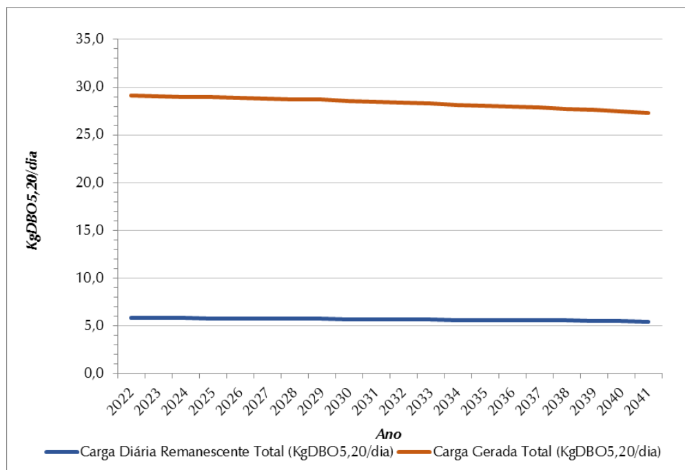
Figura 0.22 - Evolução de Cargas Orgânicas (Kg DBO 5,20 /Dia) – SES Varpa
