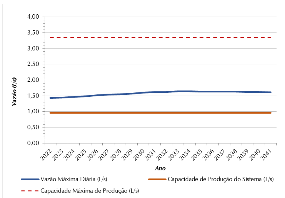
Figura 0.13 – Demandas Máximas Diárias (L/s) X Vazão Captada (L/s) – SAA Varpa
