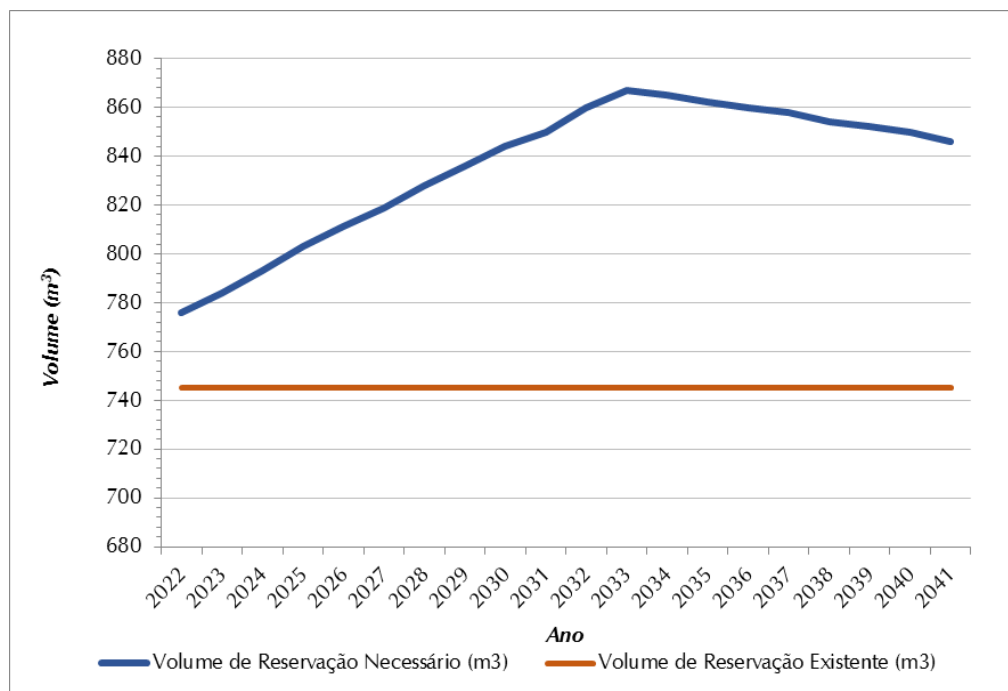
Figura 0.6 - Volume de Reservação Necessário (m³) x Volume de Reservação Atual (m³) – SAA Vila Formosa
