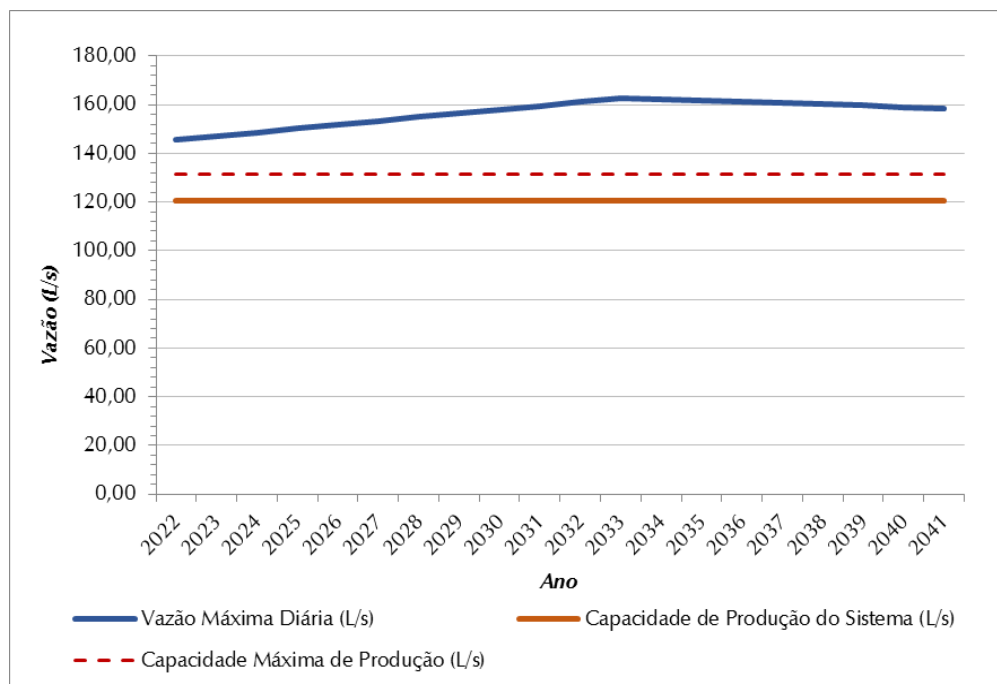
Figura 0.1 – Demandas Máximas Diárias (L/s) X Vazão Captada (L/s) – SAA Central
