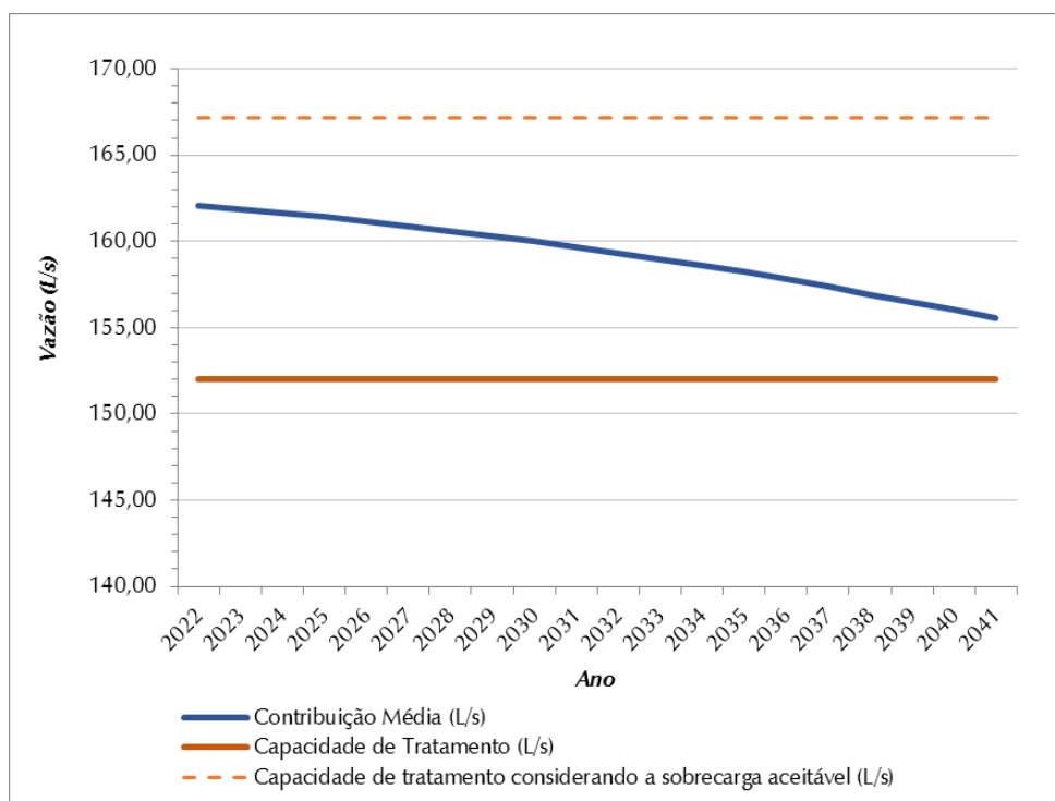
Figura 0.15 – Contribuição Média Total (L/s) x Capacidade de Tratamento de Esgoto (L/s) – SES Sede
