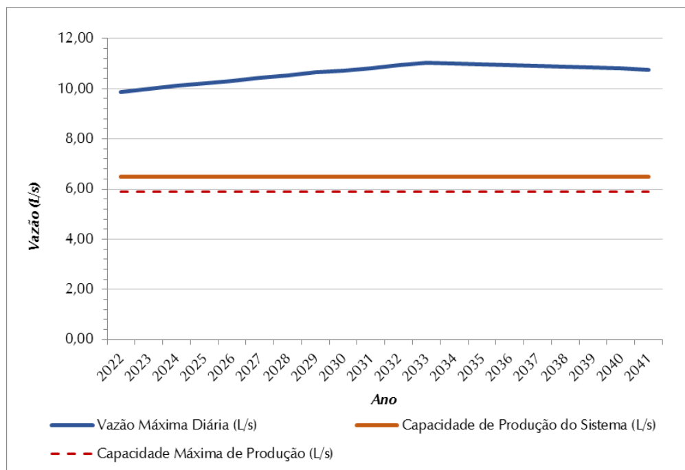
Figura 0.3 – Demandas Máximas Diárias (L/s) X Vazão Captada (L/s) – SAA Parque Universitário
