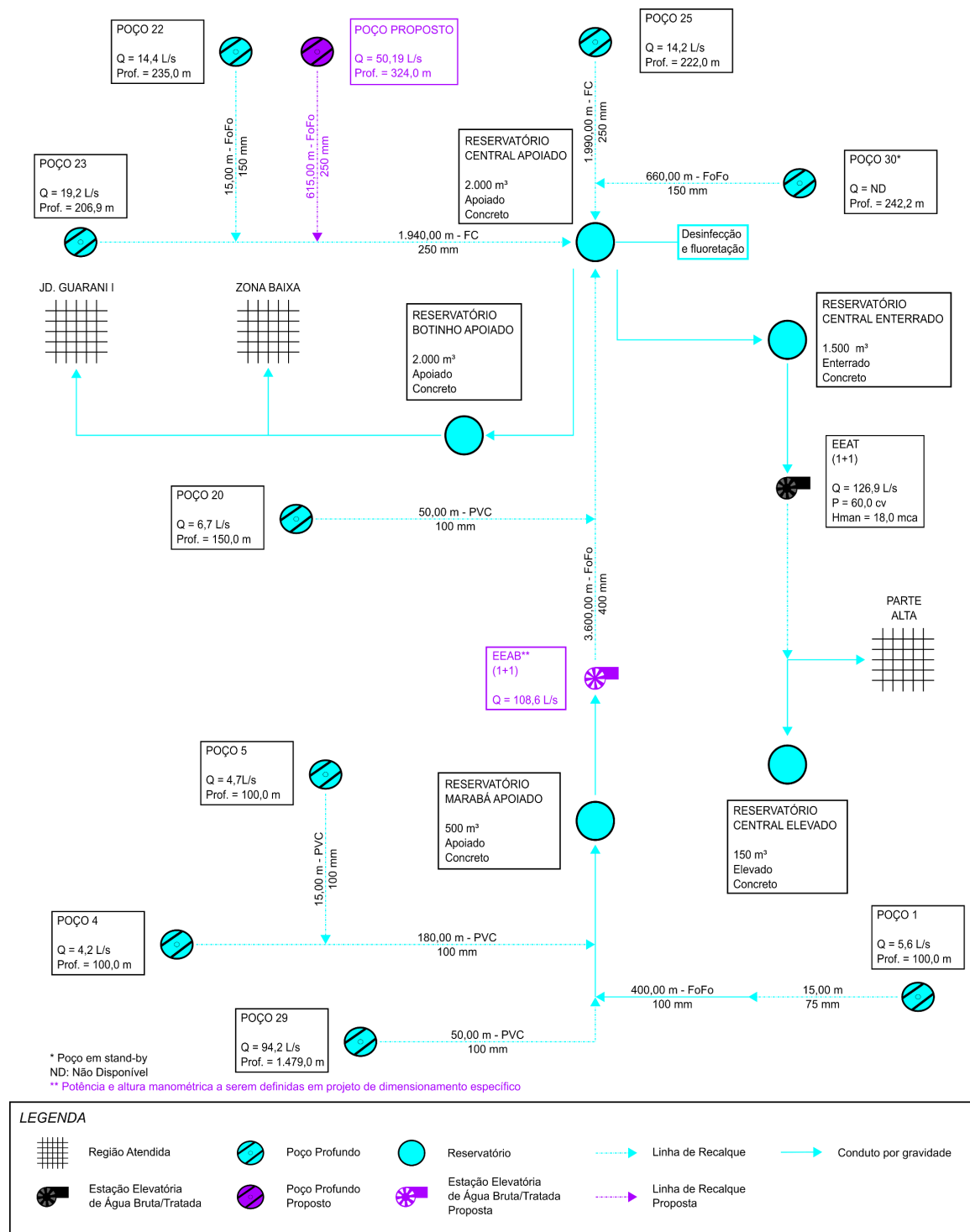
Figura 0.1 – Croqui das intervenções propostas para o sistema de abastecimento de água Central
