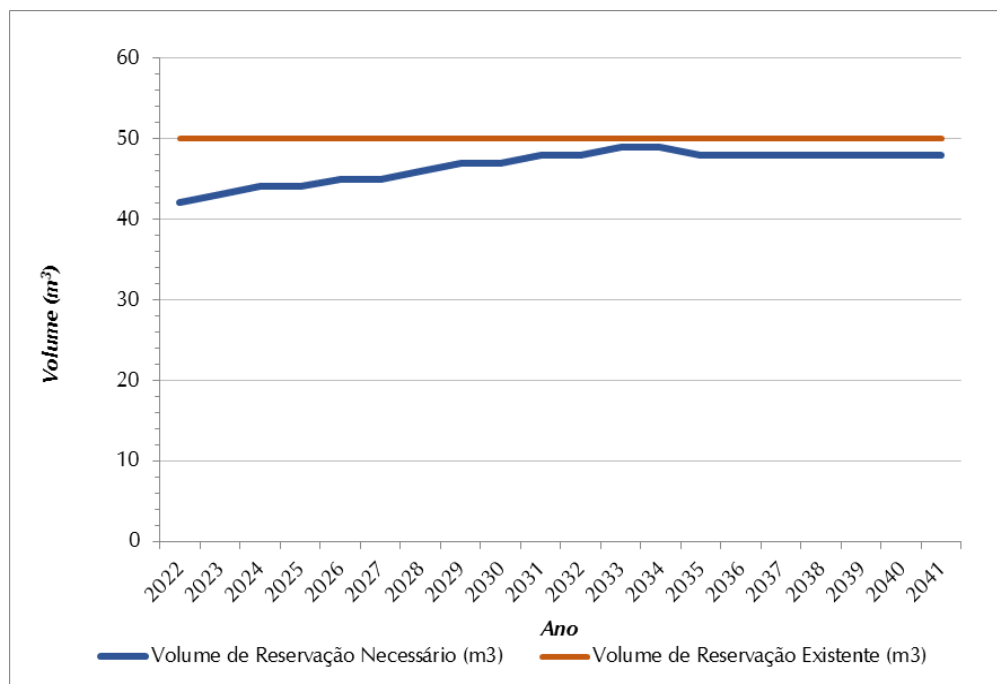
Figura 0.10 - Volume de Reserva Necessário (m³) x Volume de Reserva Atual (m³) – SAA Parnaso
