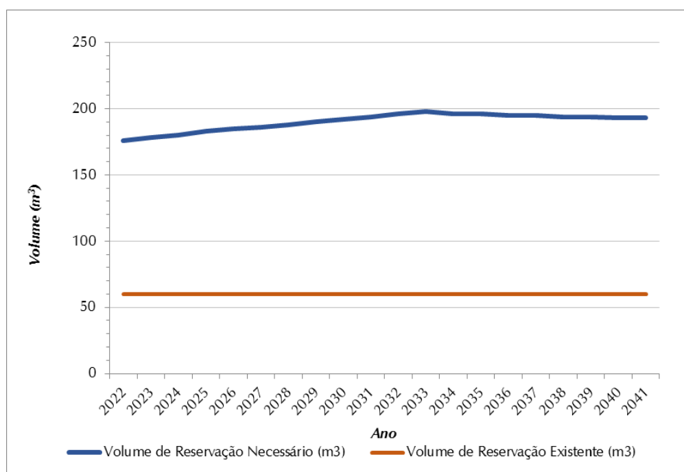
Figura 0.8 - Volume de Reservação Necessário (m³) x Volume de Reservação Atual (m³) – SAA Parque Industrial
