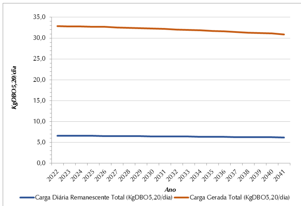
Figura 0.20 - Evolução de Cargas Orgânicas (Kg DBO 5,20 /Dia) – SES Universo
