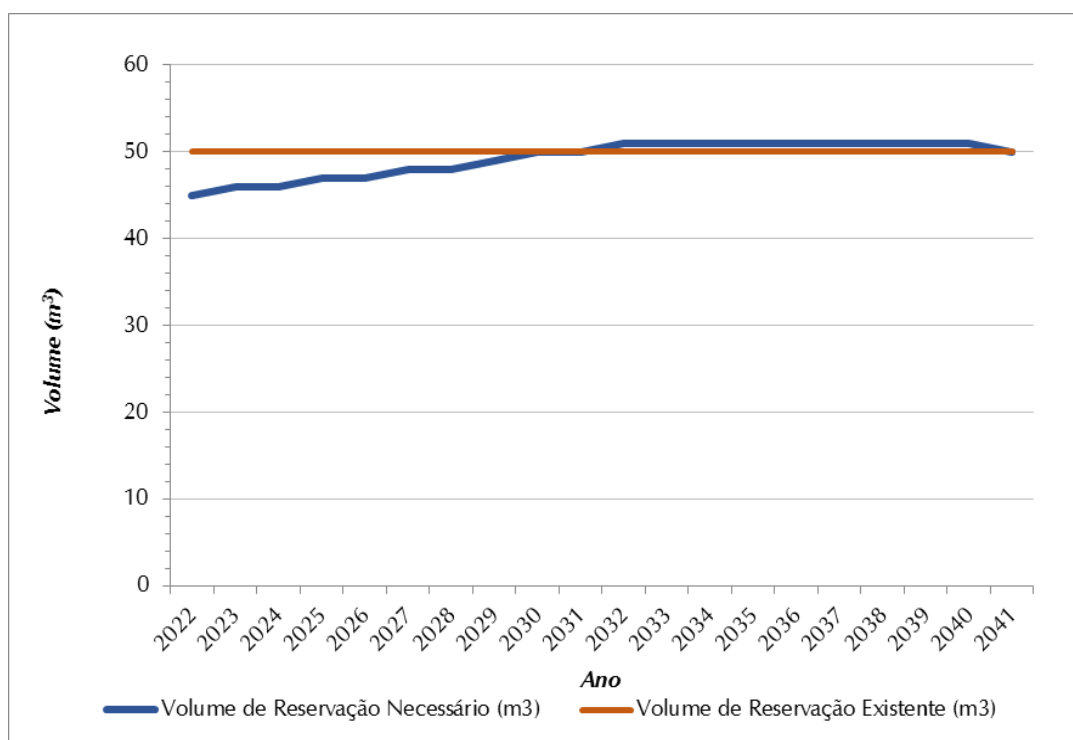
Figura 0.12 - Volume de Reservação Necessário (m³) x Volume de Reservação Atual (m³) – SAA Universo
